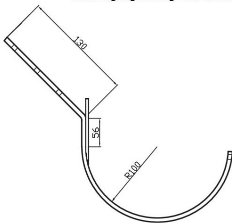
Afmetingen gootbeugel m44 met tapgat in mm.
