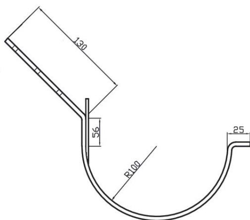
Afmetingen standaard gootbeugel m44 in mm.
